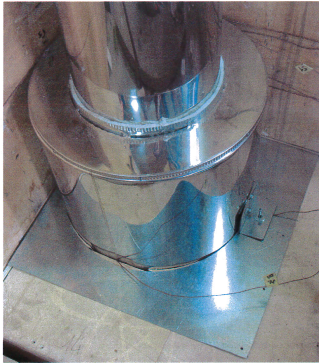
Piano superiore (con lamiera e corda fibraceramica)
