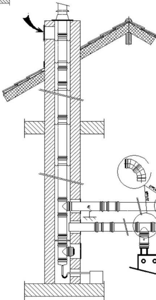
Esempi di installazione del prodotto EUROSEL
